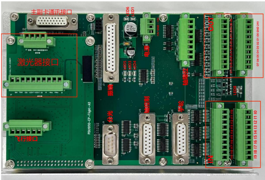
PCIE 端子板
