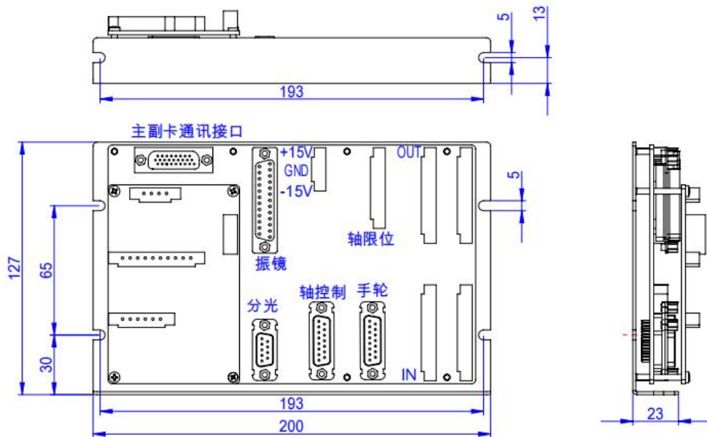
PCIE 端子板
